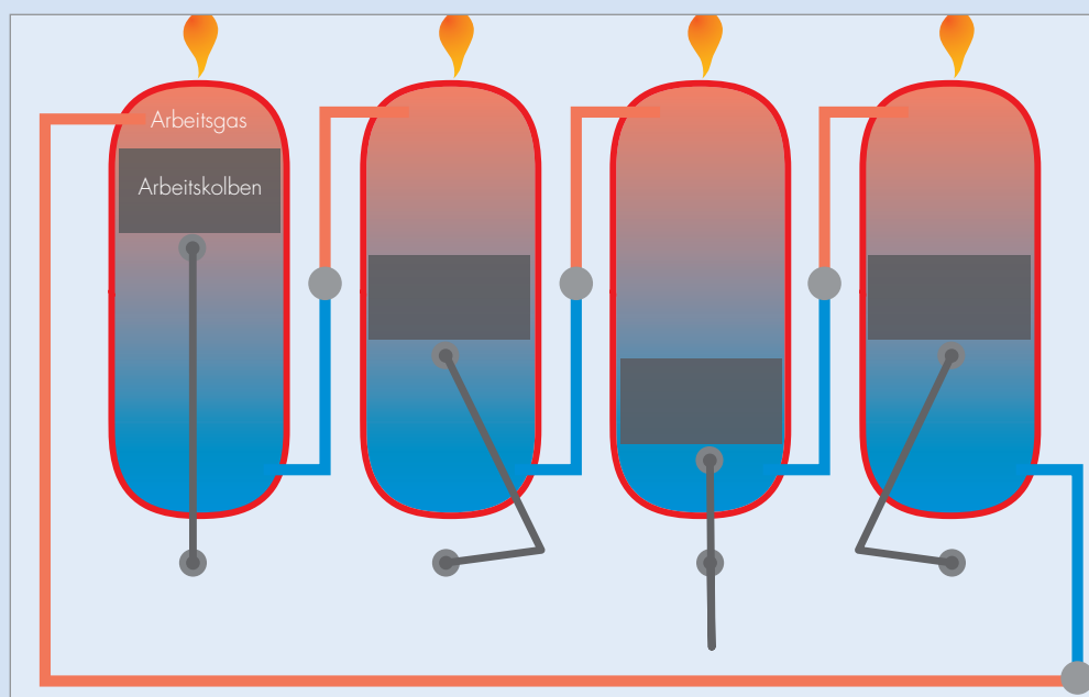
Prinzip eines 4-Zylinder-Stirlingmotors (Bauart WhisperGen)
